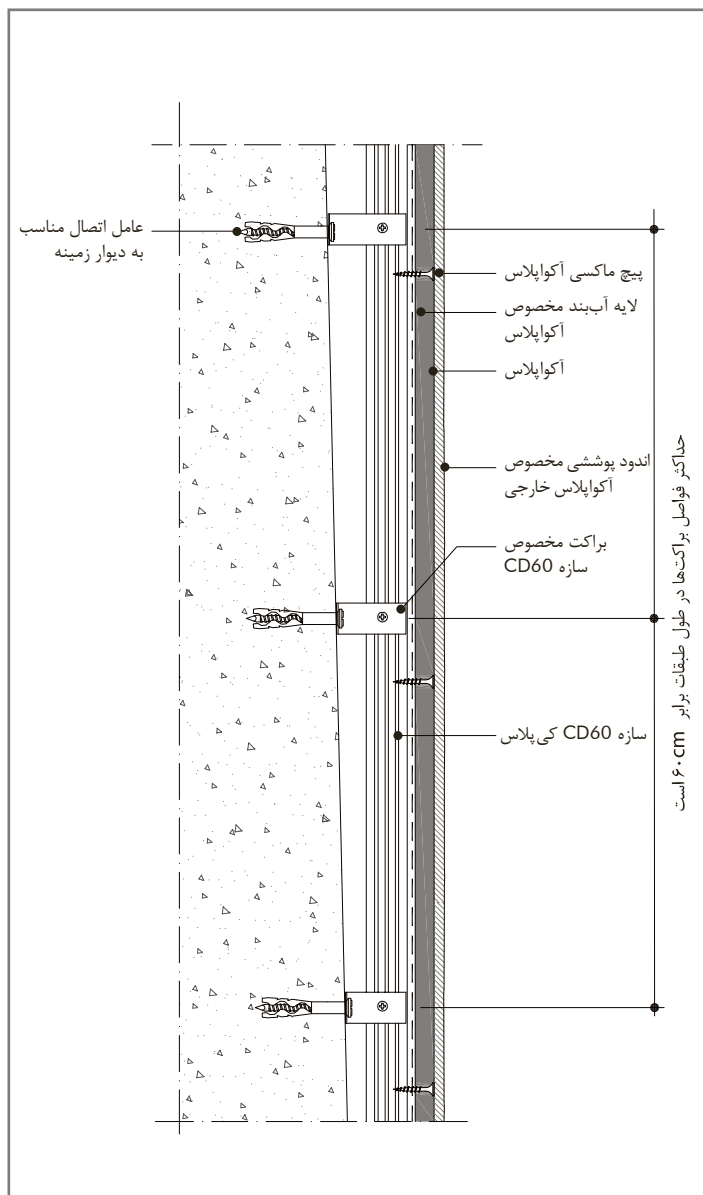
مقطع عمودی دیوار خارجی پوششی با استفاده از سازه CD60
