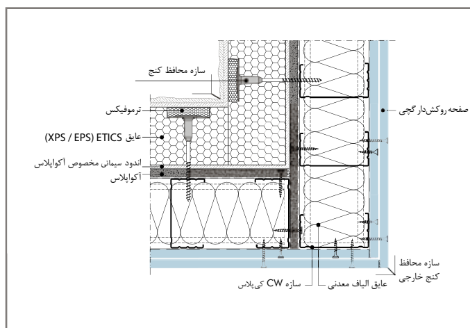
W384E - D - ETICS1: دیوار خارجی به همراه عایق الیاف معدنی و ETICS
