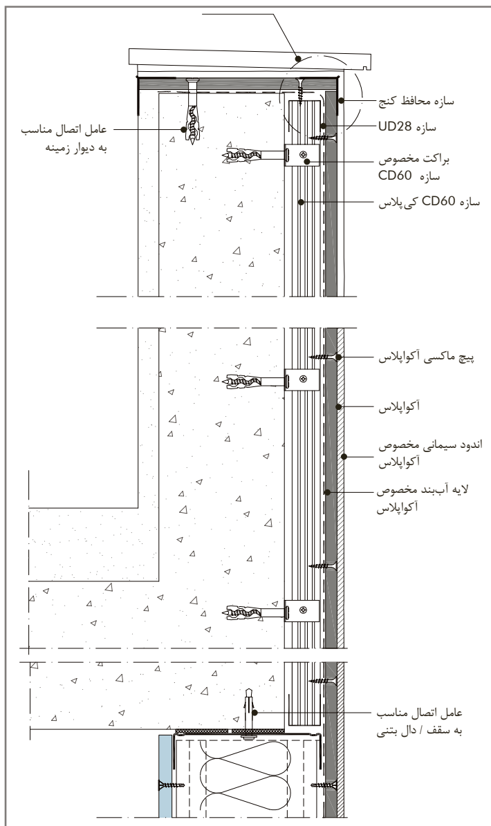
مقطع عمودی دیوار خارجی پوششی در محل جان پناه بام ساختمان با استفاده از سازه CD60
