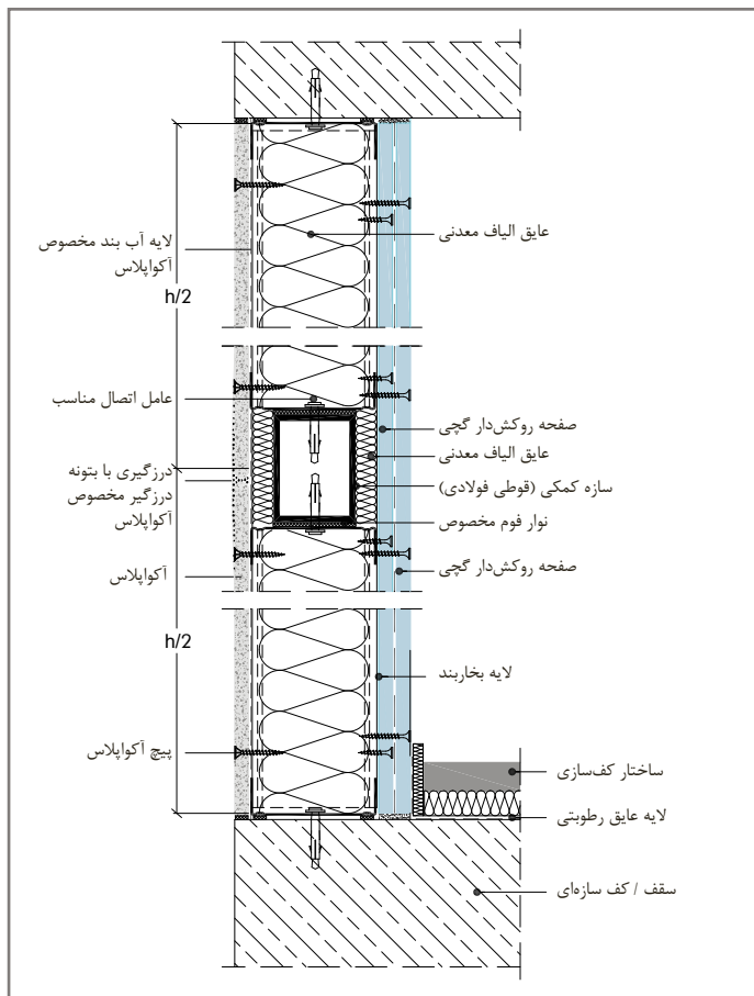
مقطع عمودی دیوار خارجی آکوپلاس با استفاده از قوطی کشی فلزی در وسط ساختار
