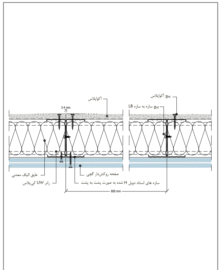
پلان دیوار خارجی آکوپلاس با استفاده از سازه استاد CW دول H
