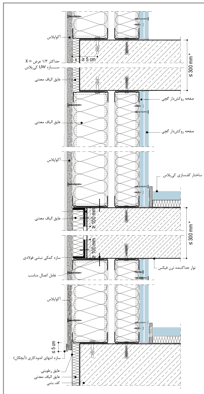
مقطع عمودی W388E-V1
