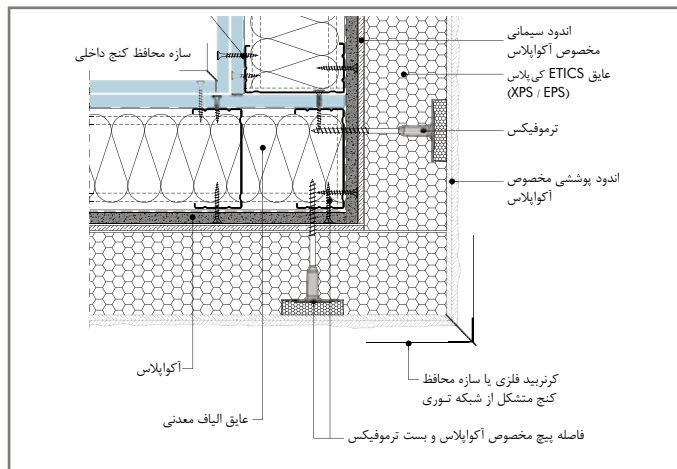
W384E - E - ETICS1: اتصال کتج خارجی با ساختار ETICS
